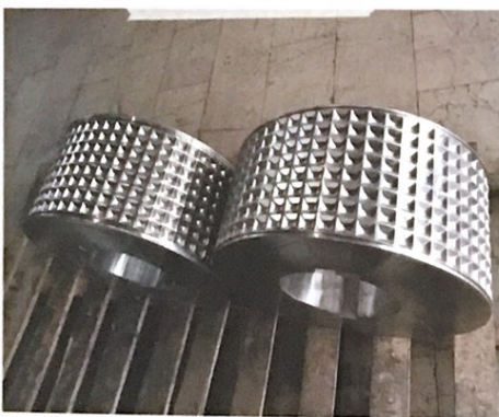
Tuz Kalıp İmalatı / Salt Mold Manufacturing
