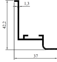
PSM-2270 Ağırlık : 0.950 kg/m
