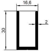
PSM-1395 Ağırlık : 2.668 kg/m
