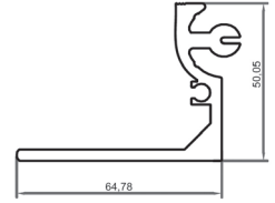
PSM-14093 Ağırlık : 0.664 kg/m
