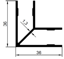
PSM-5867 Ağırlık : 1.129 kg/m
