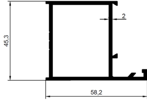
PSM-1400 Ağırlık : 1.221 kg/m
