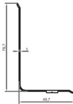
PSM-3356 Ağırlık : 1.383 kg/m
