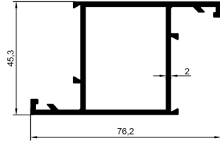
PSM-1401 Ağırlık : 0.621 kg/m
