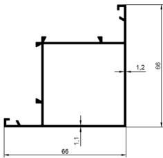
PSM-2035 Ağırlık : 0.972 kg/m
