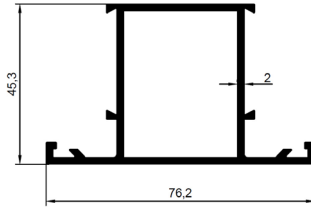
PSM-1402 Ağırlık : 4.847 kg/m
