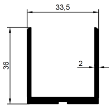
PSM-1396 Ağırlık : 0.146 kg/m
