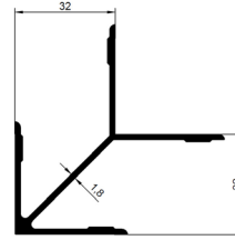
PSM-1479 Ağırlık : 0.221 kg/m
