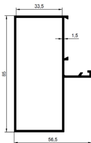
PSM-1407 Ağırlık : 1.896 kg/m
