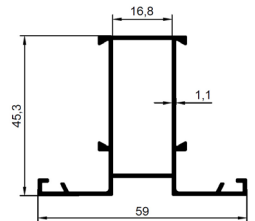
PSM-595 Ağırlık : 0.848 kg/m
