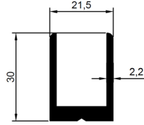
PSM-1443 Ağırlık : 0.130 kg/m
