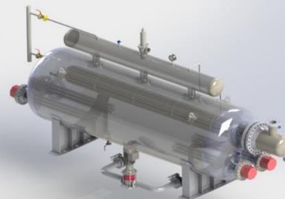
4000 Nm 3 /hr LNG Re-gasification
