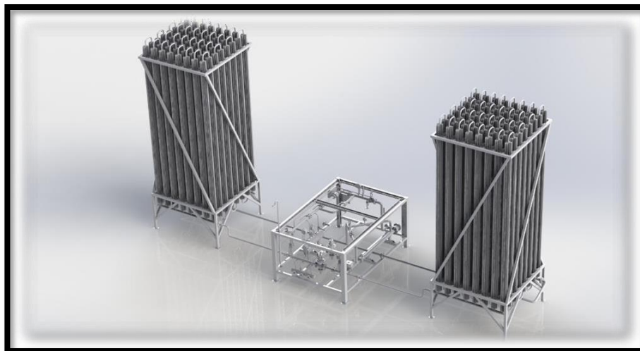
1200 Nm 3 /hr LNG Re-gasification
