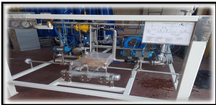
1200 Nm 3 /hr LNG Re-gasification
