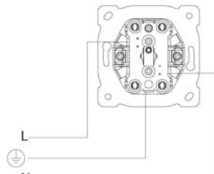
Bağlantı Şeması Connection Scheme Схема Подключения
