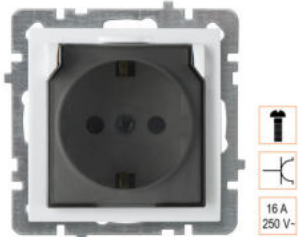
24 XX 04 20 Çocuk Korumalı Kapaklı Top. Priz Child Protected With Cover Earthed Socket Розетка с Крышкой, Зазем. и 3/Ш
