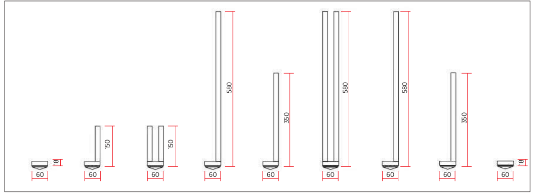
DEKOR PANELLER KESİT ÖLÇÜLERİ
