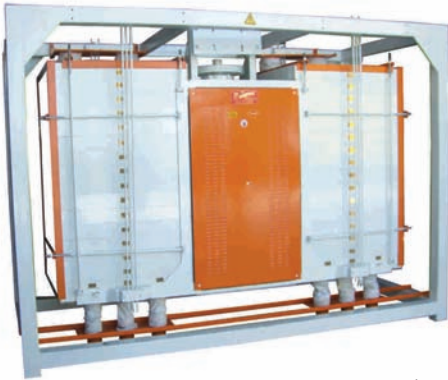
4 x 16 ELEK 4 x 16 SIEVE СИТО 4x16 غربال 4 x 16 الك 16*4 Plansichter 4 x 16
