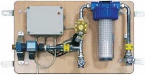
DEBİMETRE FLOWMETER ДЕБИМЕТР دبی متر دم زن نیمه اتوماتیک Débitmètre
