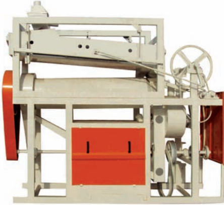
SELEKTÖR MAKİNESİ SELECTOR MACHINE СЕЛЛЕКТОРНАЯ МАШИНА ماكينة سلكتور دستگاه دانه بندی Sélecteur
