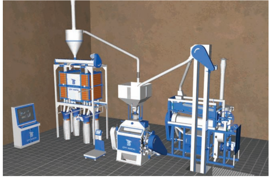
ÇK31 DİK VASLİ TESİS ÇK31 VERTICAL ROLLER MILL PLANT СК 31 МЕЛЬНИЦА С ВЕРТИКАЛЬНЫМ ВАЛЬЦОМ مصنع واليس عامودي ÇK 31 واليس عمودي CK 31 ÇK31 Usine d'Appareils Verticales
