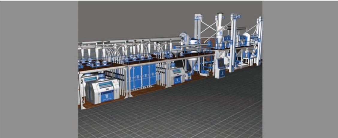
КОМПАКТНАЯ 4-Х ВАЛЬЦОВАЯ МЕЛЬНИЦА Unité compacte avec 4 Appareils a Cylindres
