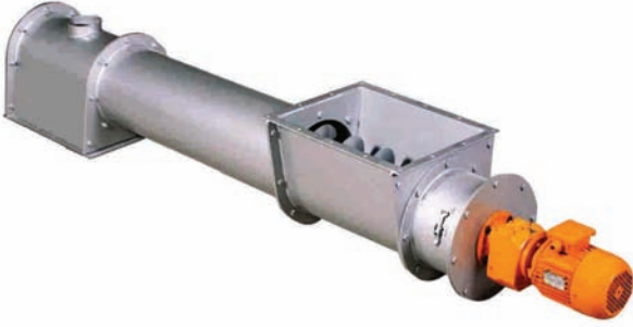
TÜP HELEZON TUBE HELIX БАЛЛОНОВЫЙ ШНЕК حلزون مغلق مارپیچ لوله ای Vis Sans Fin Type Tube
