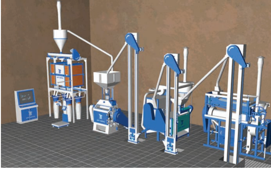
ÇK21 DİK VASLİ TESİS ÇK21 VERTICAL ROLLER MILL PLANT СК 21 МЕЛЬНИЦА С ВЕРТИКАЛЬНЫМ ВАЛЬЦОМ مصنع واليس عامودي ÇK 21 واليس عمودي CK 21 ÇK21 Usine d'Appareils Verticales
