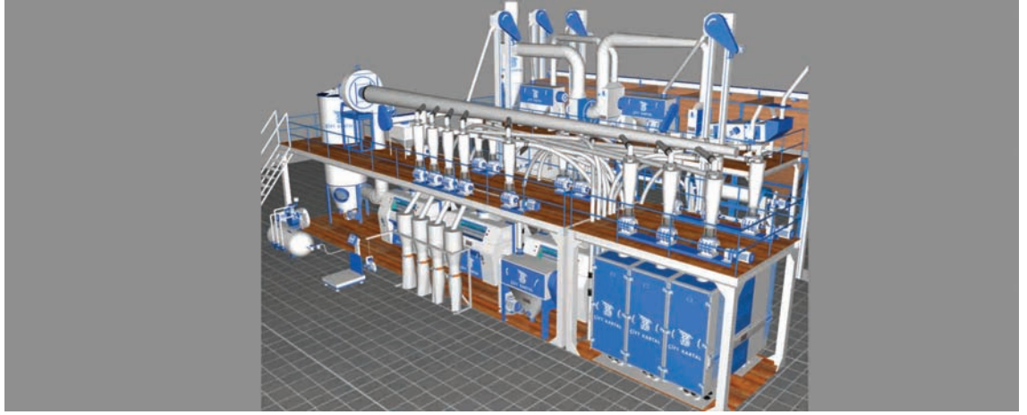
مصنع كومباكت 3 والس کارخانه آرد کامپکت 3 والسه
