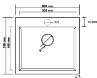
Dimensions de l'évier
