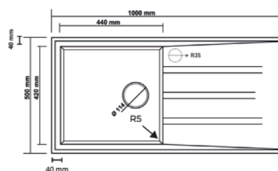
Dimensions de l'évier
