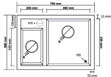
Dimensions de l'évier
