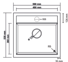
Dimensions de l'évier
