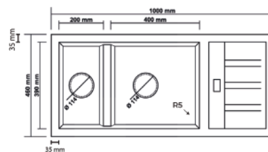
Dimensions de l'évier
