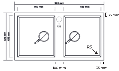
Dimensions de l'évier
