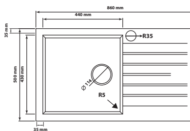
Dimensions de l'évier
