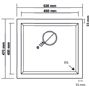
Dimensions de l'évier
