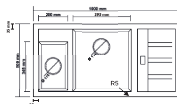
Dimensions de l'évier
