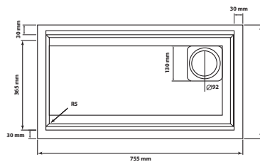
Dimensions de l'évier
