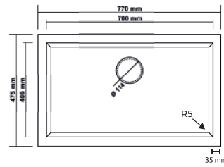
Dimensions de l'évier
