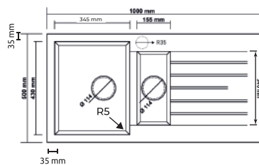
Dimensions de l'évier
