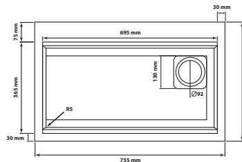
Dimensions de l'évier
