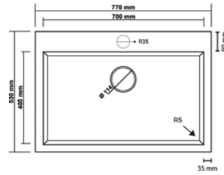
Dimensions de l'évier
