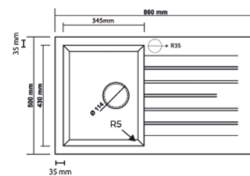
Dimensions de l'évier
