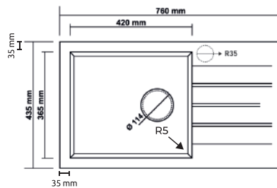
Dimensions de l'évier
