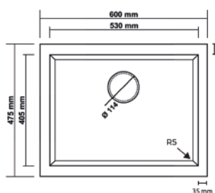
Dimensions de l'évier
